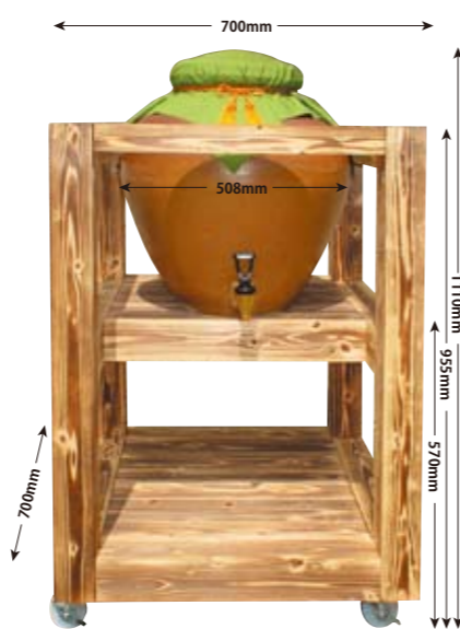
KK-54L + 専用S木製台座 (TTS-54L, TTS-90Lにも対応)
